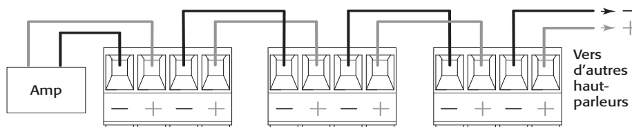
Diagramme de branchement en parallèle
